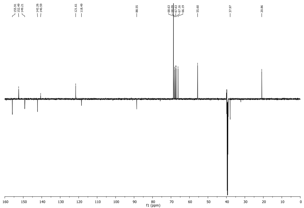
Slika 36. a) 1 H i b) 13 C NMR spektar spoja 23.
