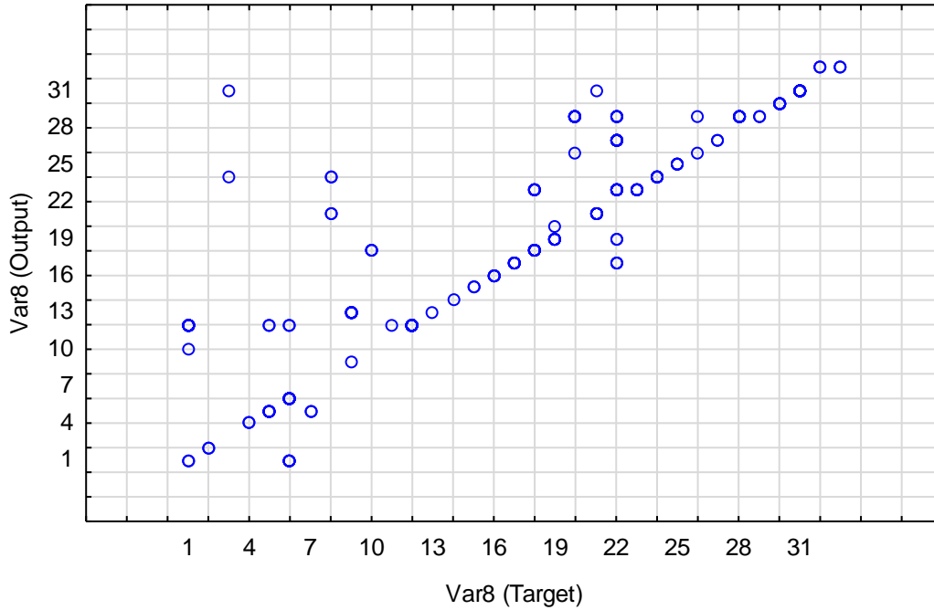
Slika 24. Točnost optimalne MLP mreže (12 neurona, eksponencijalna aktivacijska funkcija, trening funkcija padajućeg gradijenta): usporedbe modelom klasificiranih i poznatih grupiranosti uzoraka narkotika. Uspješnost predviđanja iznosi 60,66 %.
