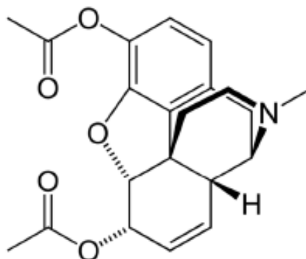
Slika 2. Struktura heroína
