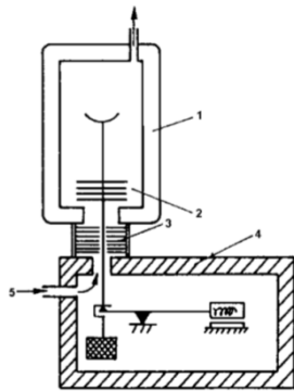
Slika 13 – Shema termovage. (1) peć, (2) zdjelica za uzorak s toplinskim štيتovima, (3) dodatna izolacija vage, (4) kućište vage, (5) ulaz inertnog plina
