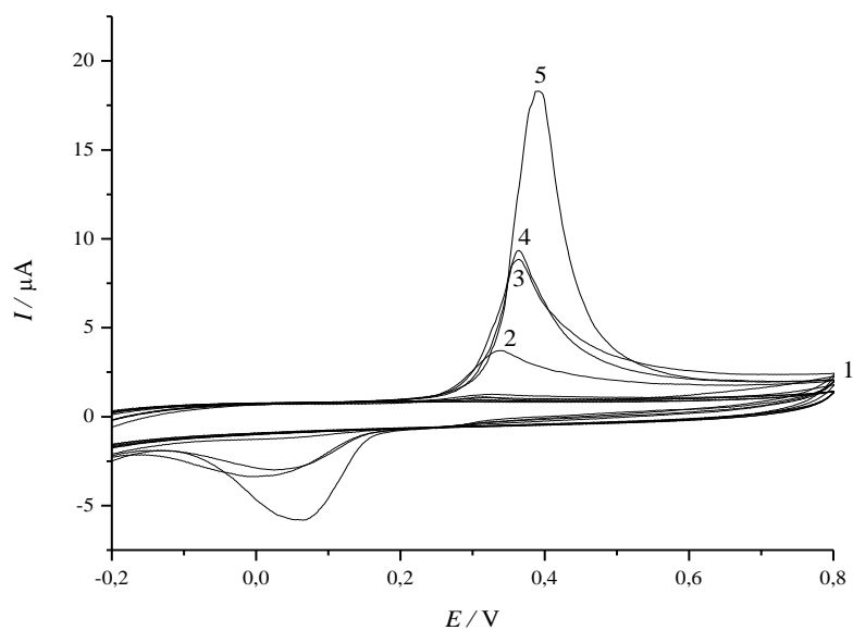
Slika 29. Ciklički voltamogrami dobiveni dodatkom 50 \mu\text{L} AgNP-PAA tinte u 10 mL BR pufera u rasponu pH vrijednosti 10,00 – 6,00. Taloženo s 0,01 M \text{H}_2\text{C}_2\text{O}_4 . 1 – BR puferi pH = 10,00 – 8,00 ; 5 – pH = 6,00; 4 – pH = 6,50; 3 – pH = 7,00; 2 – pH = 7,50.
