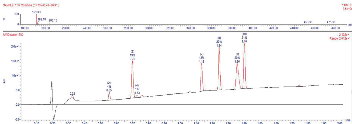
Slika 27. Profil Buchwald-Hartwigove reakcije grijane uz pomoć mikrovalnog zračenja praćen na UPLC s UV i masenim detektorima.
