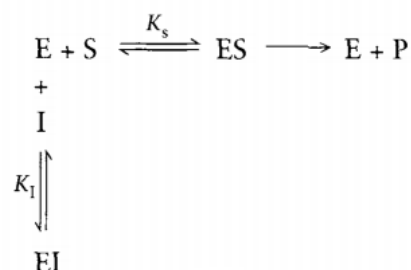
Slika 2.13. Shematski prikaz kompetitivne inhibicije.
