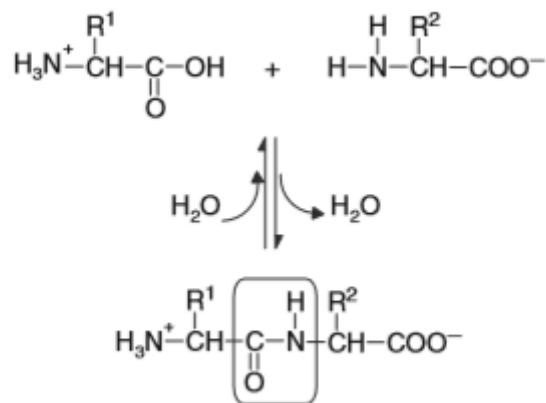
Slika 2.2. Nastajanje peptidne veze između dvije \alpha -aminokiseline.
