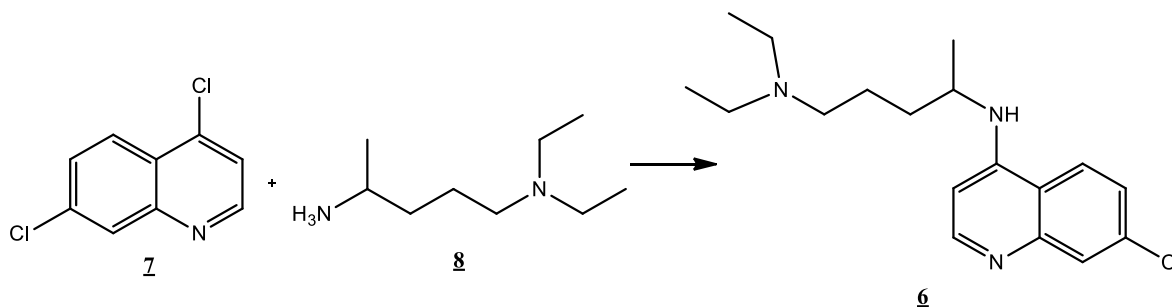
Shema 1. Sinteza klorokina
