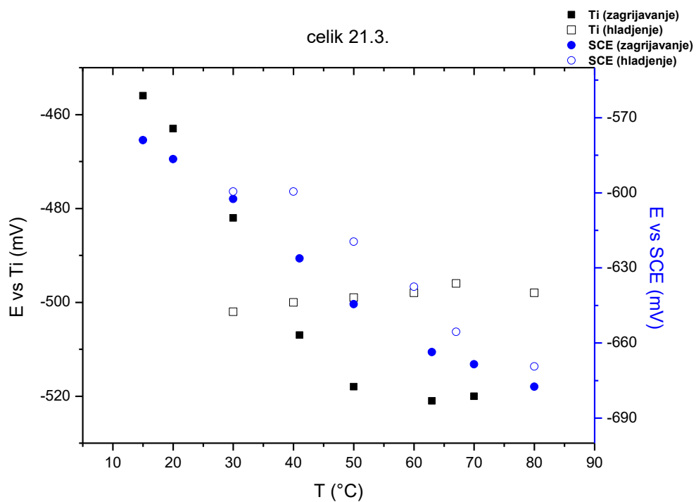
Slika 34. Ovisnost korozijskog potencijala o temperaturi za uzorak ugljičnog čelika koristeći Ti kao pseudo-referentnu elektrodu (puni znakovi -zagrijavanje, prazni znakovi - hladjenje)
