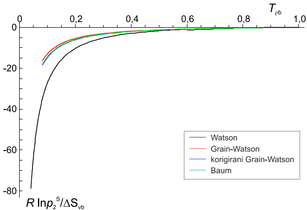
Slika 3.2. Ovisnost ravnotežnog tlaka sublimacije o reduciranoj temperaturi, T_{\rho b} .
