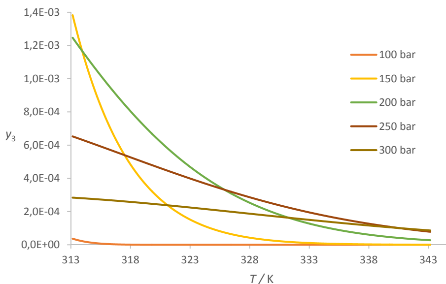
Slika 3.4. Izobare topljivosti nimbina u smjesi \text{CO}_2 i etanola, sastava (0,99 : 0,005)
