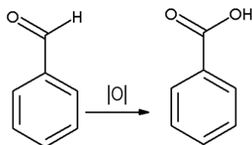
Shema 4. Oksidacija benzaldehida
