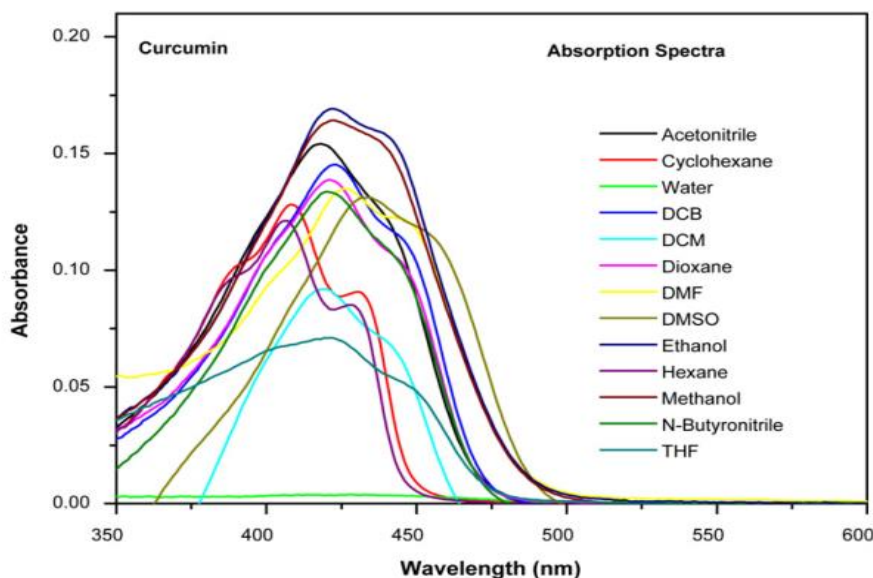
Slika 7. Apсорpcijski spektar kurkumina u različitim otapalima, pri sobnoj temperaturi [3].
