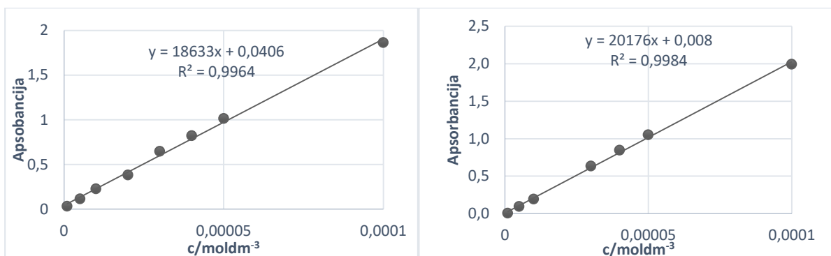
Slika 107. (lijevo) Kalibracijska krivulja miricetina u otopini etanola pri maksimumu apsorpcije od 377,89 nm
