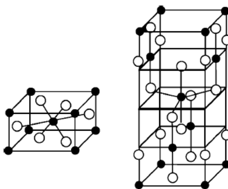
Slika 1. Shema kristalnih struktura rutila (lijevo) i anatasa \text{TiO}_2 (desno)
