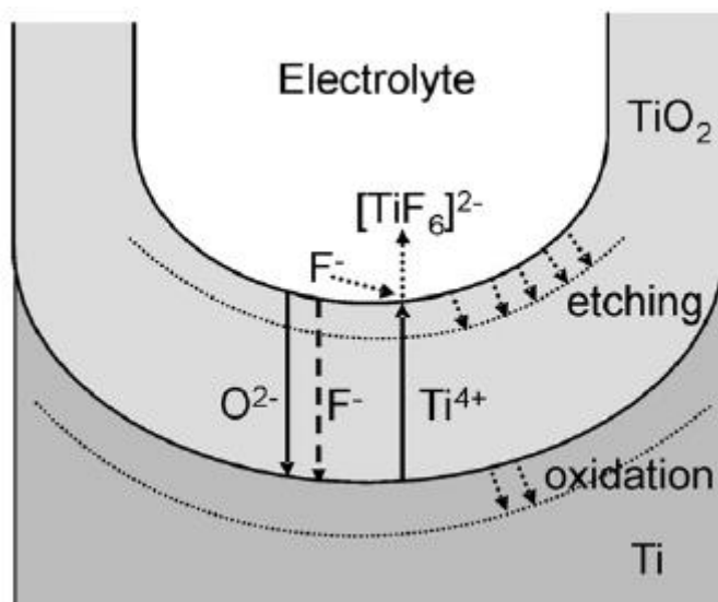
Slika 2. Shematski prikaz anodizacije Ti u prisutnosti fluorida
