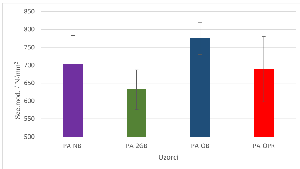
Slika 40 Grafički prikaz promjene sekantnog modula ( E ) pretaljane uzorke PA 12
