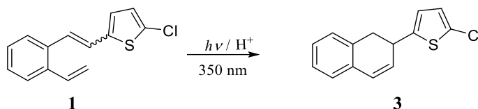
Shema 2.4.
