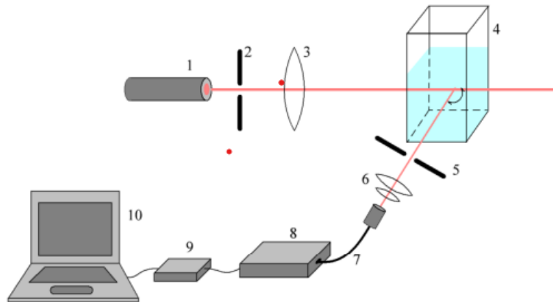
Slika 2-12. Shema DLS uređaja
