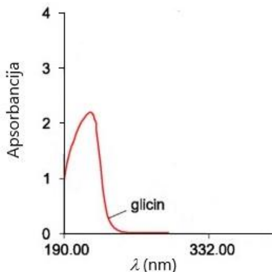
Slika 23. UV/VIS spektar molekule glicina
