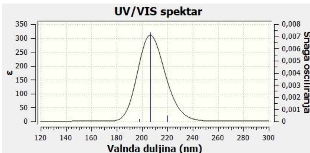
Slika 24. Dobiveni UV/VIS spektar molekule glicina
