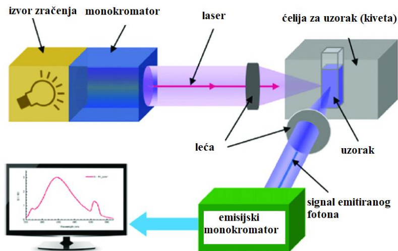
Slika 6. Shema spektrofiorimetra
