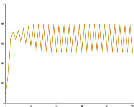
Slika 3.2. Generacijski prikaz i paukova mreža logističkog preslikavanja za \lambda = 3.2
