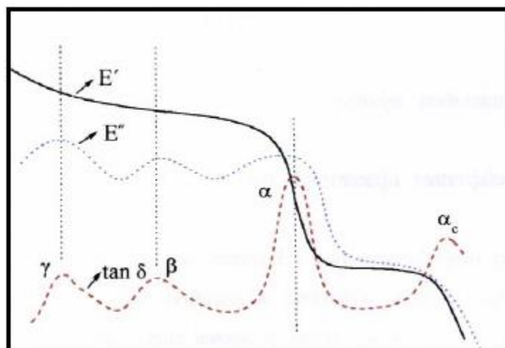
Slika 19. Prikaz tipičnog DMA spektra amorfne polimera [15].
