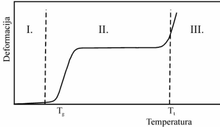
Slika 5. Termomehanička krivulja linearnog amorfno polimera (I staklasto, II viskoelastično ili kaučukasto, III viskofluidno ili kapljevitostanje) [7].
