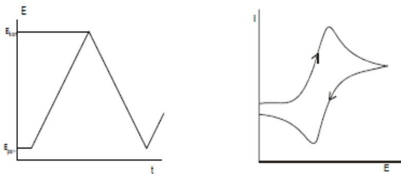
Slika 2.12. Signal pobude (lijevo) i signal odziva (desno) u cikličkoj voltometriji 19
