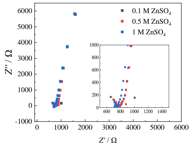
Slika 4.9. Nyquistov prikaz ovisnosti imaginarne o realnoj komponenti impedancije za rGO/ 20 % AC elektrodu
