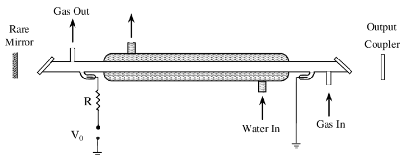
Slika 14. Shema \text{CO}_2 lasera [4]
