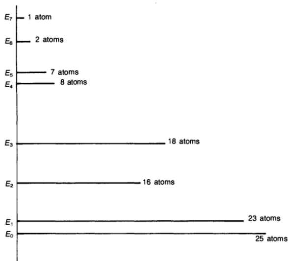
Slika 5. Inverzija napučenosti [1]
