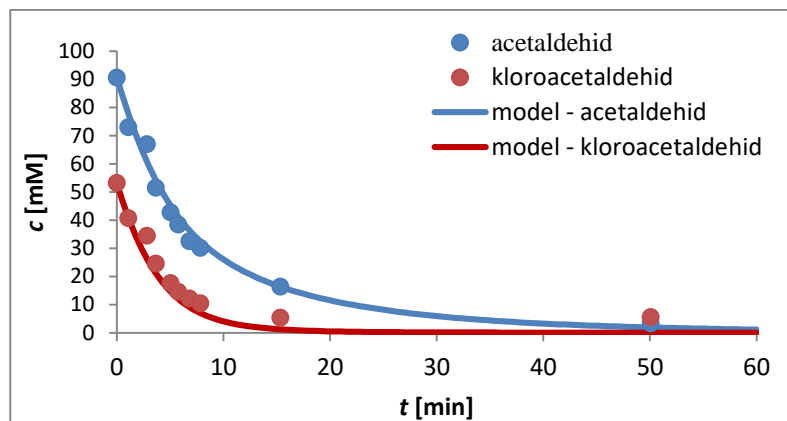
Slika 28. Sinteza 6-kloro-3,5-dihidroksiheksanala aldolnom adicijom katalizirana enzimom DERA u kotlastom reaktoru (0,1 M fosfatni pufer pH 6 , \gamma_{\text{DERA}} = 3 \text{ mg cm}^{-3} , c_{\text{AA}} = 90,76 \text{ mM} , c_{\text{CAA}} = 53,27 \text{ mM} ). Vremenska promjena koncentracije supstrata.
