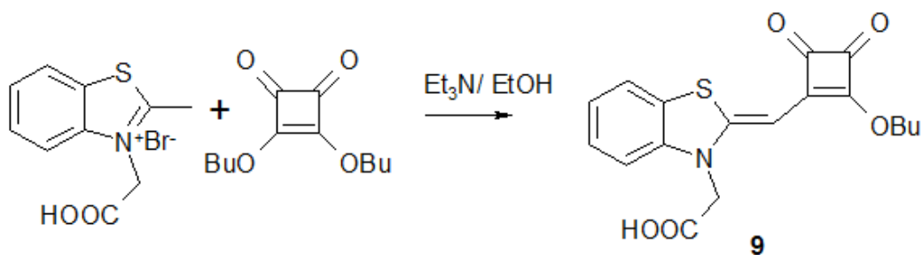
Slika 27. Sinteza spoja 9 [23].
