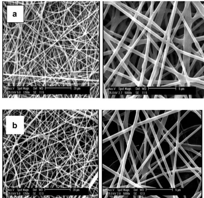
Slika 2.14. Slika nanovlakana kefran/PVA dobivena SEM mikroskopom u različitim udaljenostima mlaznice od kolektora: (a) 120, (b) 150.
