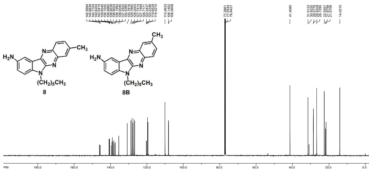
Slika 30. 13 C NMR spektar (CDCl 3 ) smjese 8 i 8B
