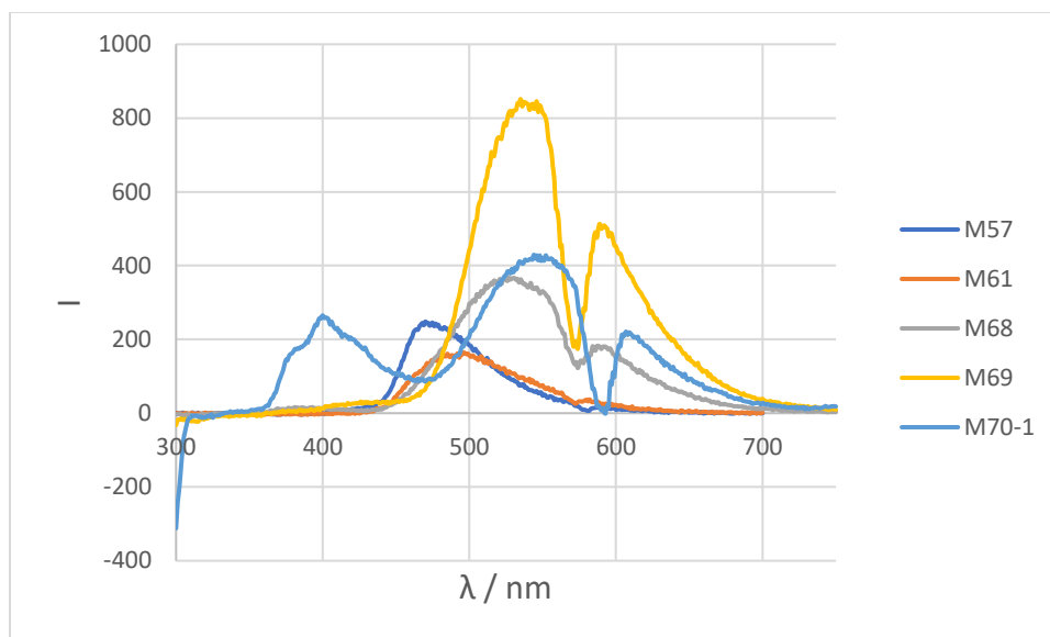
SLIKA 30: Usporedba emisijskih spektara zaštićenih gvanidina
