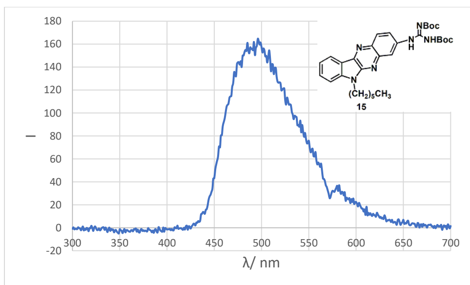
Slika 74. Emisijski spektar ( \text{CH}_3\text{CN} ) spoja 15
