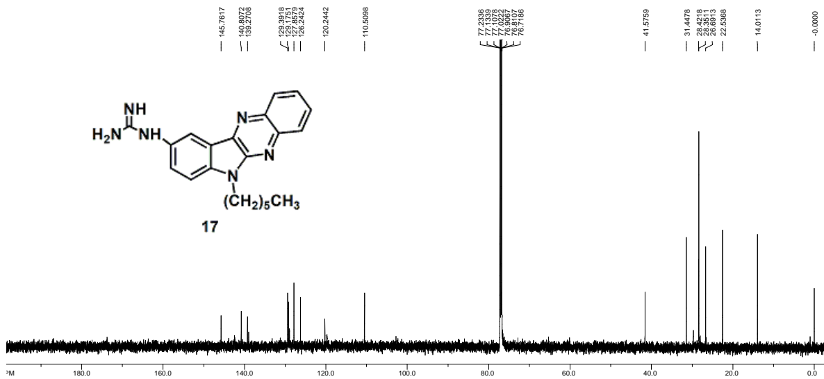
Slika 20. 13 C NMR spektar (CDCl 3 ) spoja 17
