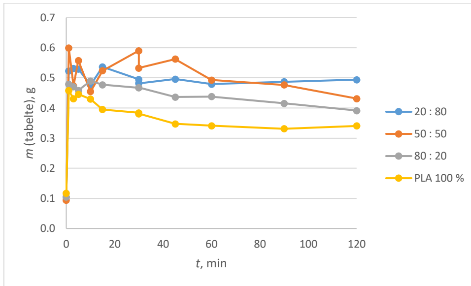
Slika 24. Srednja promjena mase tableta u vremenu
