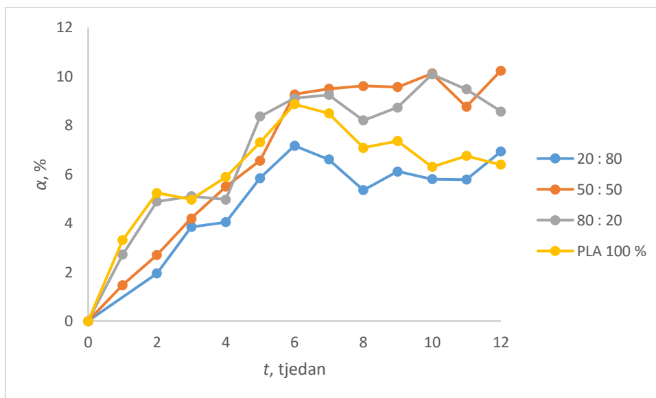
Slika 25. Grafički prikaz procesa bubrenja
