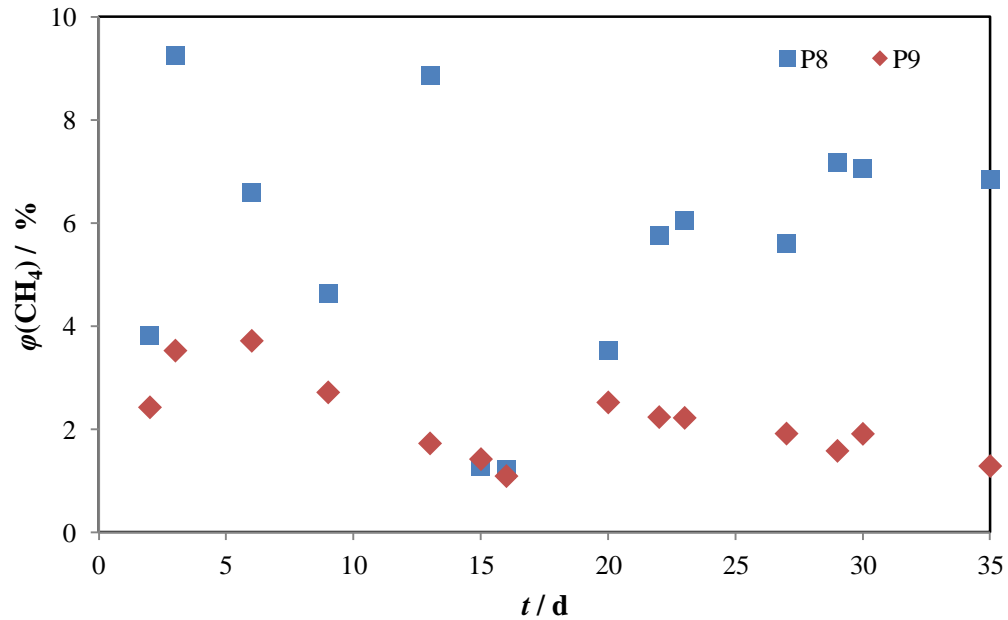
Slika 4.11. Volumni udio metana u bioplina u pokusima P8 i P9.
