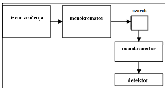
Slika 11. Shema fluorimetra
