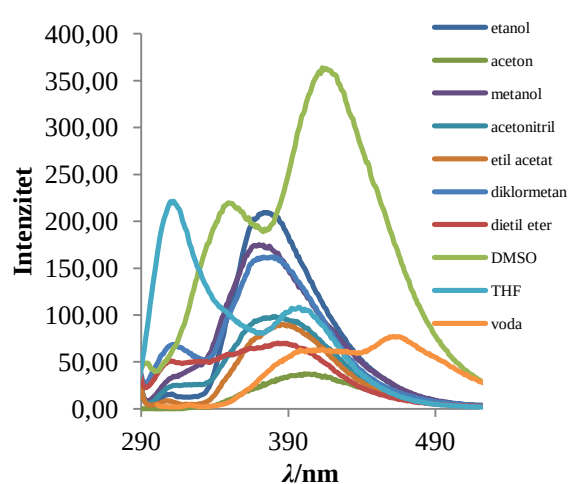
Slika 23. a) apsorpcijski spektar; b) emisijski spektar spoja 4 u različitim otapalima snimljeni u istim eksperimentalnim uvjetima
