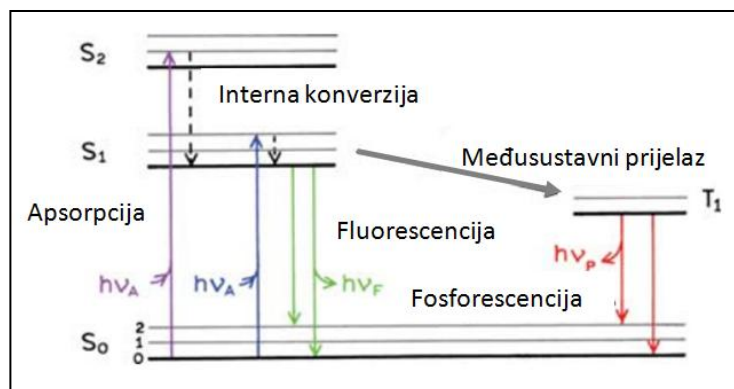
Slika 10. Jablonski dijagram
