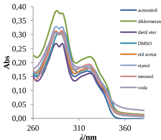
Slika 24. a) apsorpcijski spektar; b) emisijski spektar spoja 5 u različitim otapalima snimljeni u istim eksperimentalnim uvjetima
