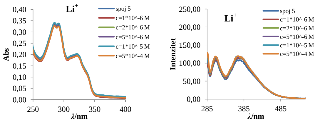
Slika 26. Apsorpcijski i emisijski spektri različitih koncentracija metalnih iona a) \text{Cu}^{2+} ; b) \text{Hg}^{2+} ; c) \text{Zn}^{2+} ; d) \text{Al}^{3+} ; e) \text{Fe}^{3+} ; f) \text{Ca}^{2+} ; g) \text{Ag}^{+} i h) \text{Li}^{+} za spoj 5, c = 1 \cdot 10^{-5} M
