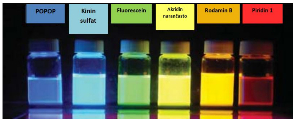
Slika 9. Prikaz struktura fluoroforma i njihovih boja
