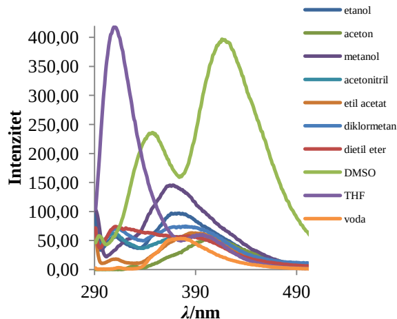
Slika 24. a) apsorpcijski spektar; b) emisijski spektar spoja 5 u različitim otapalima snimljeni u istim eksperimentalnim uvjetima
