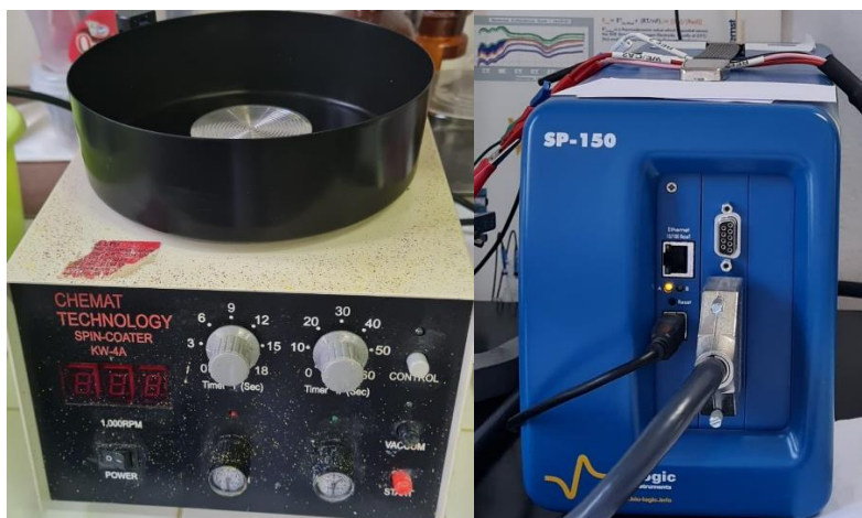
Slika 3.3. Spin-coater korišten za imobilizaciju fotokatalizatora na supstrat (lijevo); potencijostat (desno)
