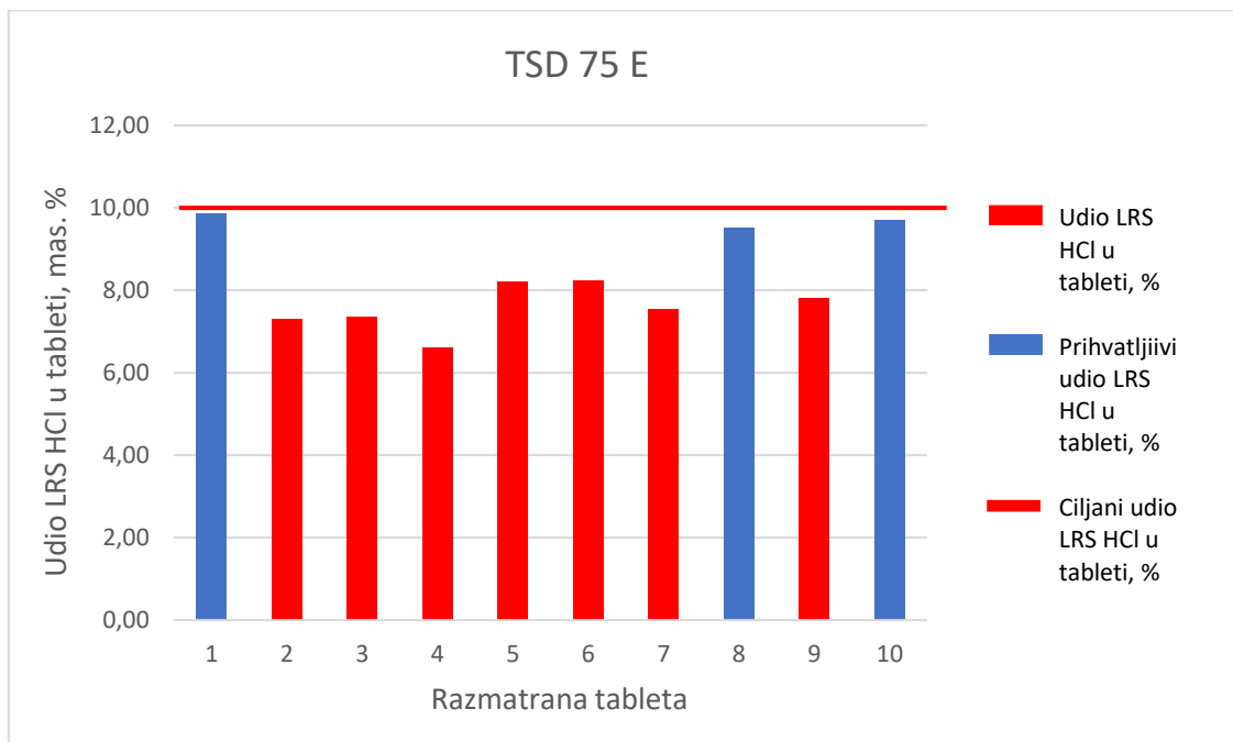
Slika 5.10. Sadržaj lurasidon-hidroklorida u tabletama uzorka TSD 75 E.
