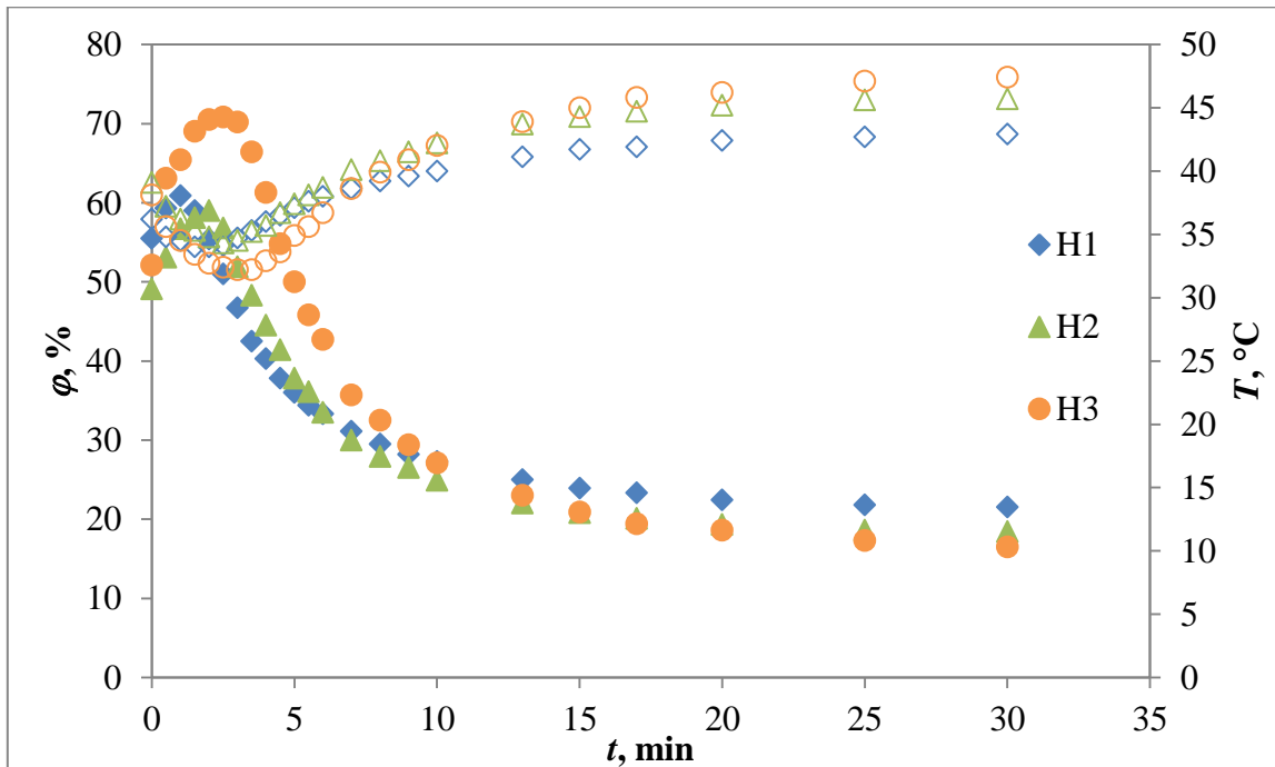
Slika 11. Eksperimentalni podaci na izlazu iz sušionika: temperatura i relativna vlažnost za tri različite visine sloja čestica ( T=60\text{ }^\circ\text{C} i v = v_2\text{ m/s} )
