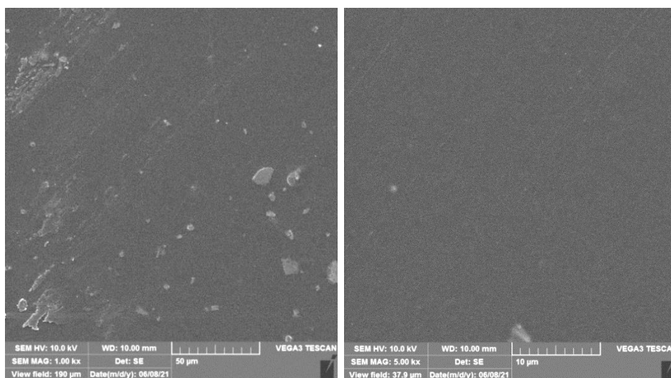
Slika 4.5. SEM mikrografi uzorka polimernog filma kitozana (Cs) pri povećanju od 1000 (lijevo) i 5000 (desno) puta
