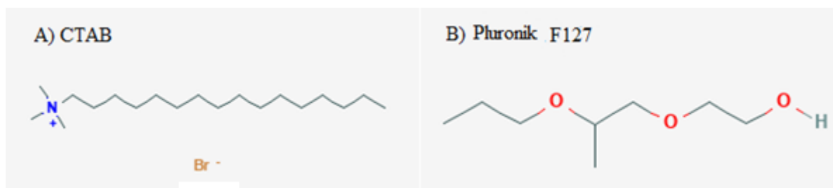
Slika 10. Strukturne formule surfaktanta A) CTAB [29] i B) Pluronik F127 [30]
