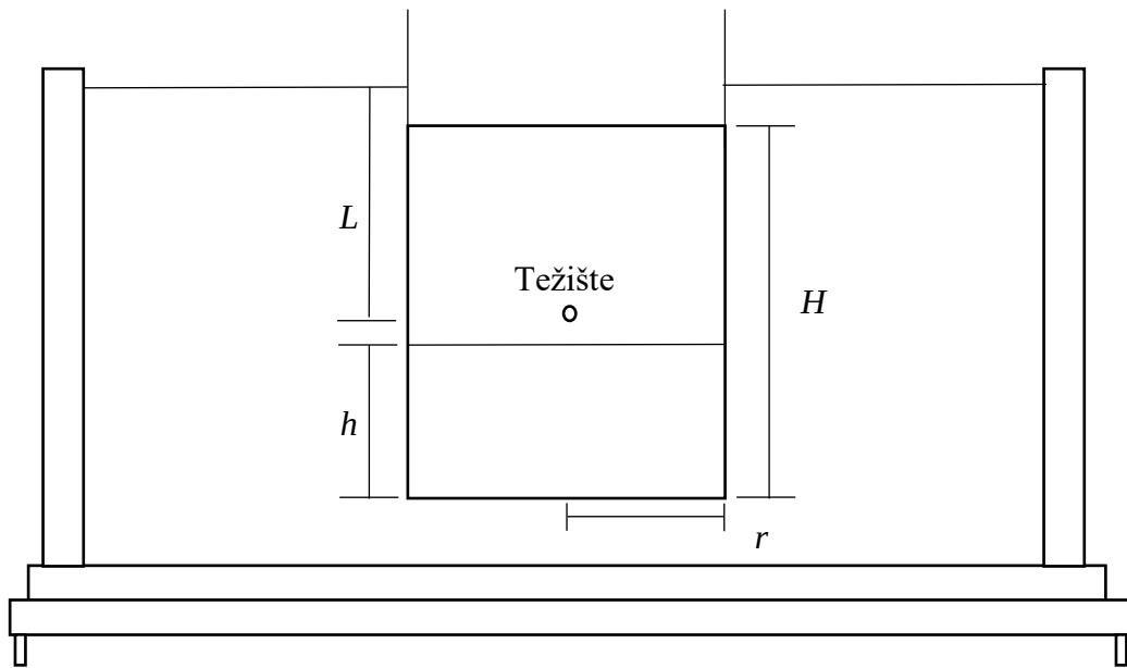
Slika 5. Shematski prikaz fizičkog njihala, uz izvod vlastite kružne frekvencije nosača uzorka i valjkastog uzorka.
