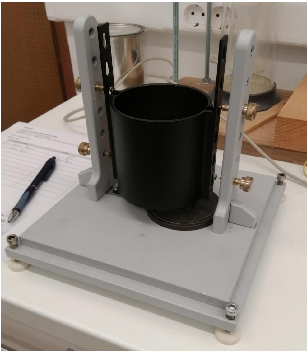
Slika 6. Fotografija aparature.
