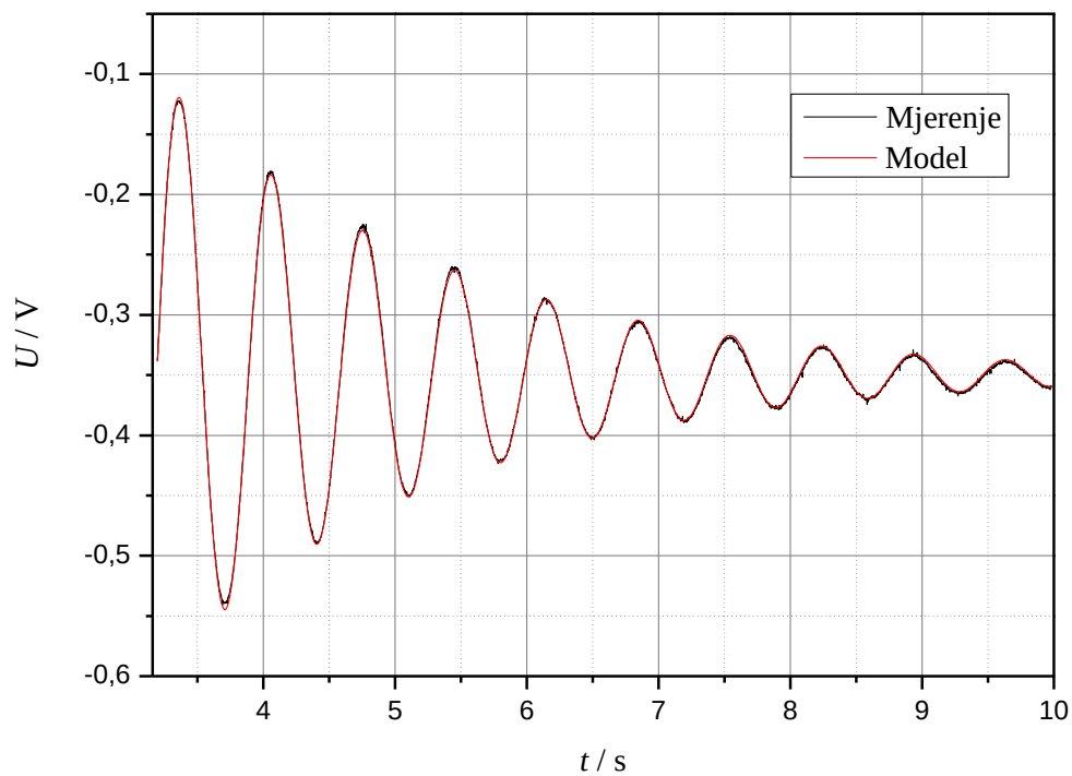
Slika 9. Utočnjavanje mjernih podataka titranja posude oko prve osi rotacije.
