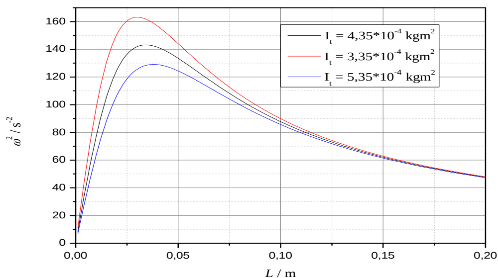
Slika 15. Prikaz utjecaja različitih vrijednosti momenta inercije prazne posude oko osi rotacije koja prolazi kroz njeno težište na krivulju ovisnosti kvadrata kružne frekvencije o udaljenosti težišta prazne posude od osi rotacije. Model je prikazan korištenjem jednadžbe (25).
