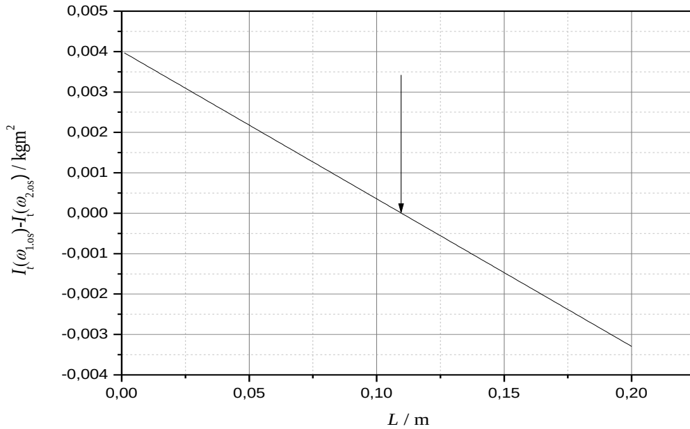
Slika 4. Grafički postupak određivanja udaljenosti osi titranja od težišta tijela. Masa fizičkog njihala je m=0,37082 kg, \omega_1^2 = 81,0 s -2 , \omega_2^2 = 100,0 s -2 , ubrzanje sile teže je g=9,80662 ms -2 .
