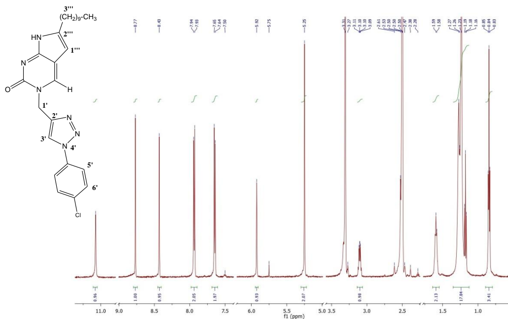
Slika 7. 1 H NMR spektar spoja 23
