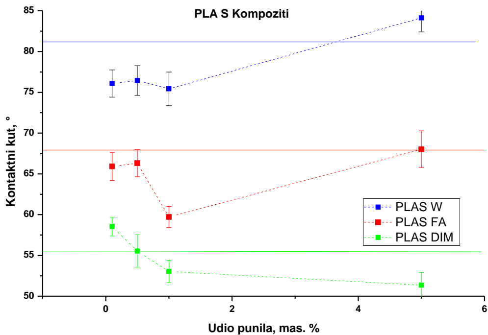
Slika 4.35. Kontaktni kutevi testnih kapljica na uzorcima kompozita PLA S
