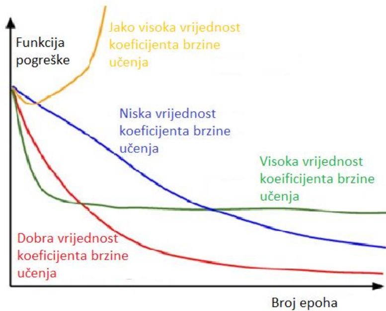
Slika 12. Utjecaj vrijednosti koeficijenta brzine učenja na treniranje mreže [20]
