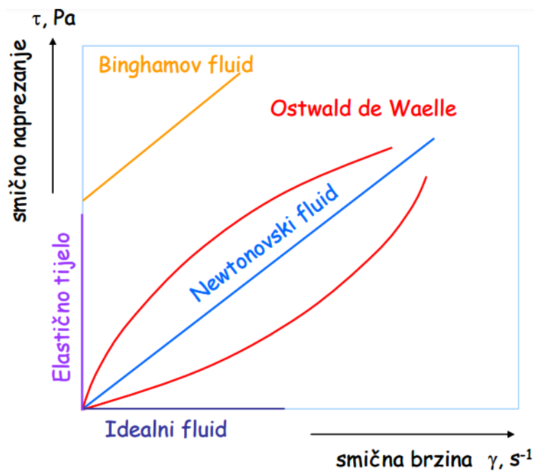
Slika 4. Reološki dijagram 16
