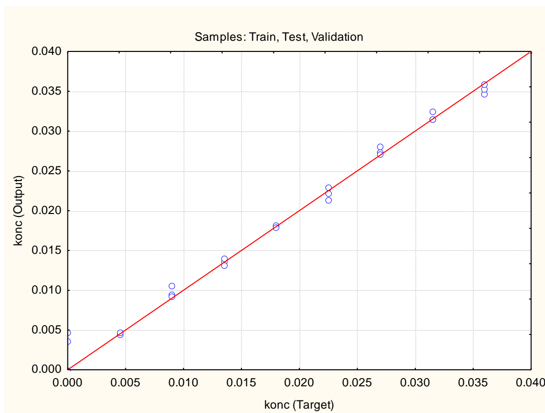
Slika 11. Korelacija predviđanja koncentracije glicerola izabrane neuronske mreže i eksperimentalnih vrijednosti
