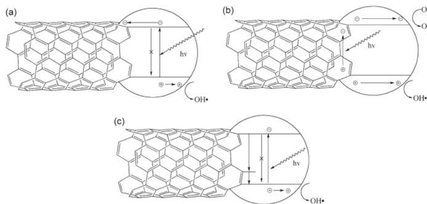
Slika 5.: Mehanizmi poboljšanja fotokatalitičke aktivnosti \text{TiO}_2 pomoću ugljikovih nanocijevi: a) CNT djeluju kao elektron-akceptori i onemogućuju brzu rekombinaciju elektrona i šupljina, b) Foton u CNT generira par elektronskih rupa, te na temelju relevantnih položaja vrpce, elektron (ili šupljina) injektira se u vodljivu vrpću \text{TiO}_2 stvarajući radikale \text{O}_2^{\bullet-} ili \text{OH}^{\bullet} , c) Oksidirane ugljikove nanocijevi mogu djelovati kao nečistoća kroz \text{Ti-O-C} veze [19]
