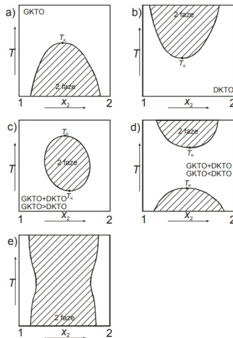
Slika 4. Različiti oblici ovisnosti ravnotežnih sastava kapljevitih faza o temperaturi. a) mješljivost kapljevina raste s povišenjem temperature, kritična točka nalazi se iznad dvofaznog područja. b) mješljivost se smanjuje s povišenjem temperature. c) sustav sa zatvorenom petljom mješljivosti i dvjema kritičnim temperaturama. d) sustav s dvjema kritičnim temperaturama, najbolja mješljivost pri srednjoj temperaturi. e) sustav koji nema potpune mješljivosti.
