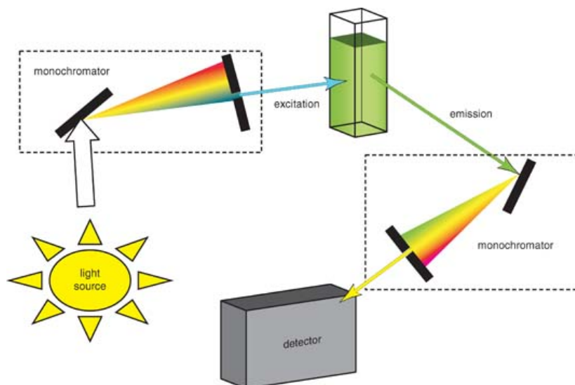
Slika 12. Shematski prikaz fluorescentnog spektrometra
