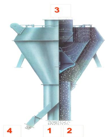
Slika 4. Separator sirovine
