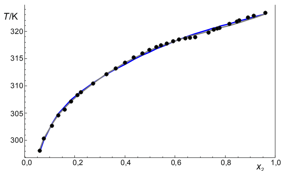
Slika 21. Ovisnost ravnotežne temperature taljenja o množinskom udjelu za sustav metil- tert -butil-eter (1) – n -tetrakozan (2) za troparametarski (tamnoplavi) i četveroparametarski (sivi) Redlich-Kisterov model
