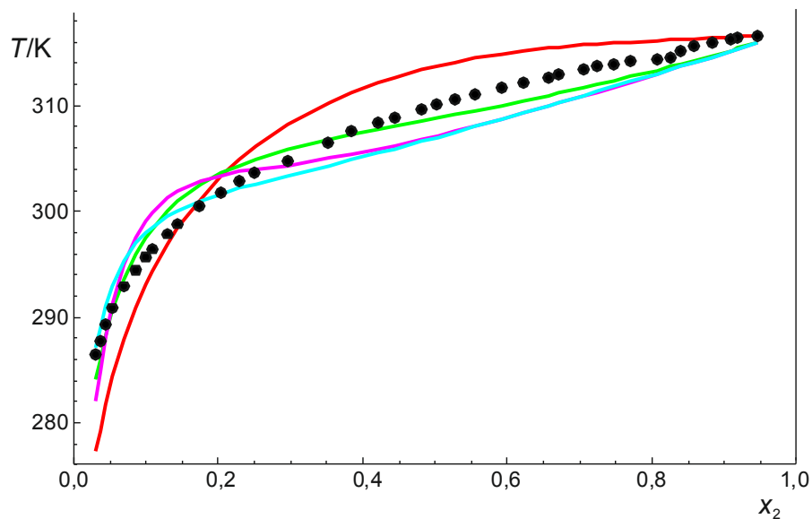
Slika 20. Ovisnost ravnotežne temperature taljenja o množinskom udjelu za sustav metil- tert -butil-eter (1) – n -dokozan (2) za Wilsonov model (crvena), te modele NRTL (zeleni), UNIQUAC (ružičasti) i UNIFAC (svijetloplavi).
