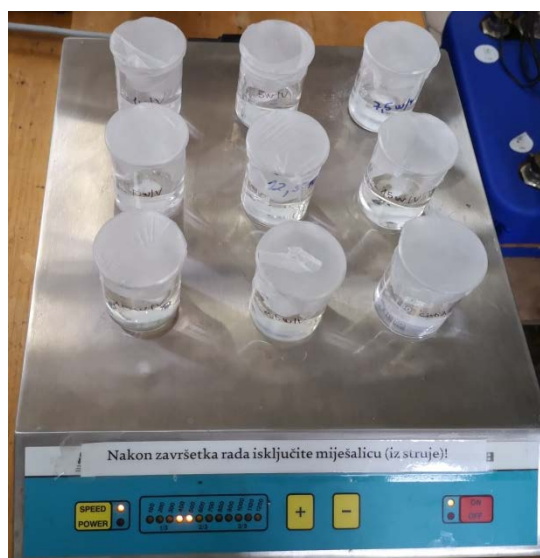
Slika 4.6. Fotografija uzorka LRS HCl u otopini pufera s odgovarajućim polimerom na magnetskoj miješalici
