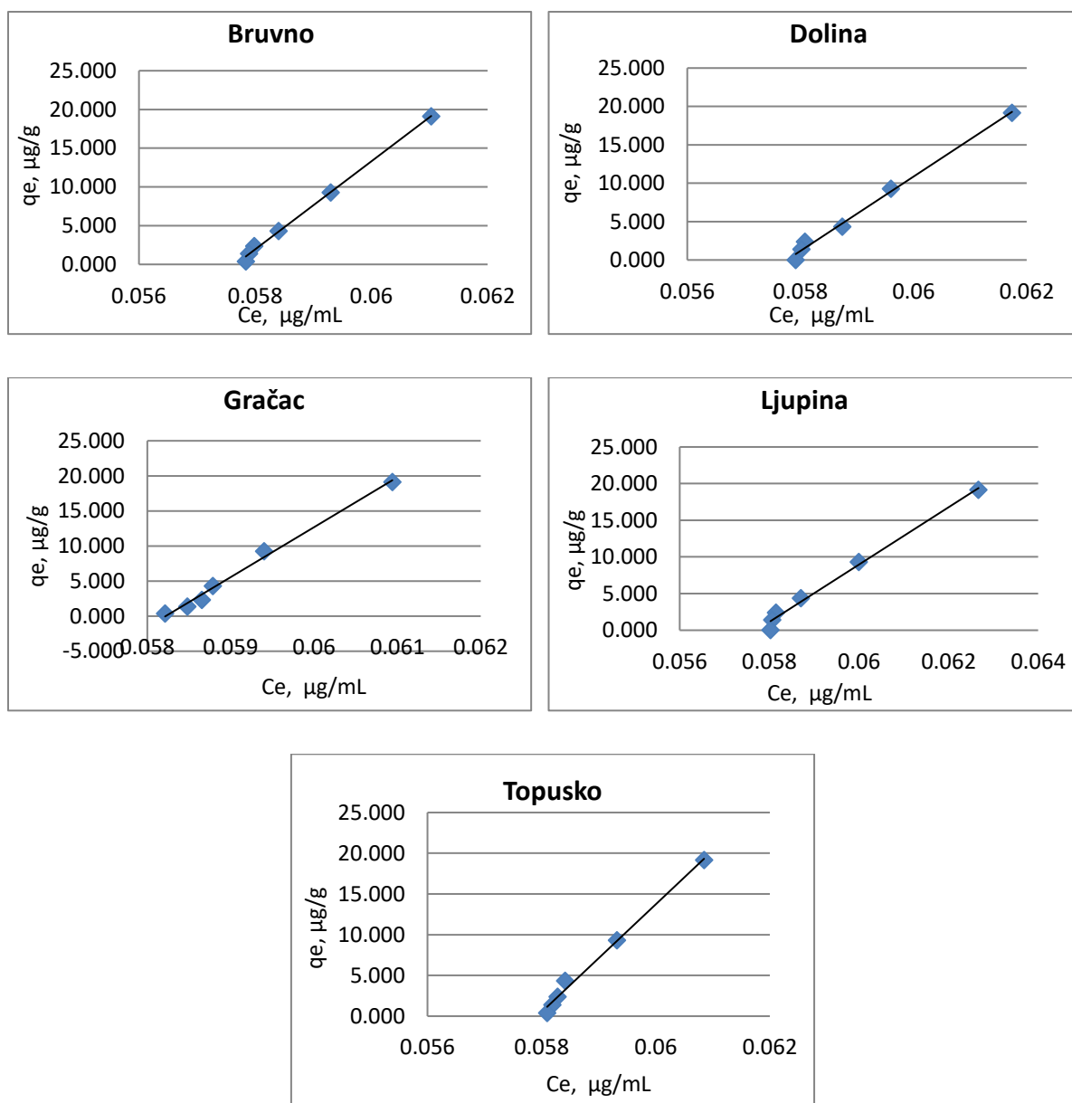
Slika 4.9. Grafički prikaz linearnih desorpcijskih izoterami hidroklorokina za ispitivana tla u otopini 0,01 M \text{CaCl}_2 pri početnoj pH vrijednosti
