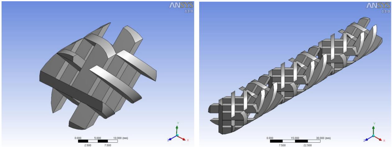
(a) Jedan CSE-X4 element za miješanje
