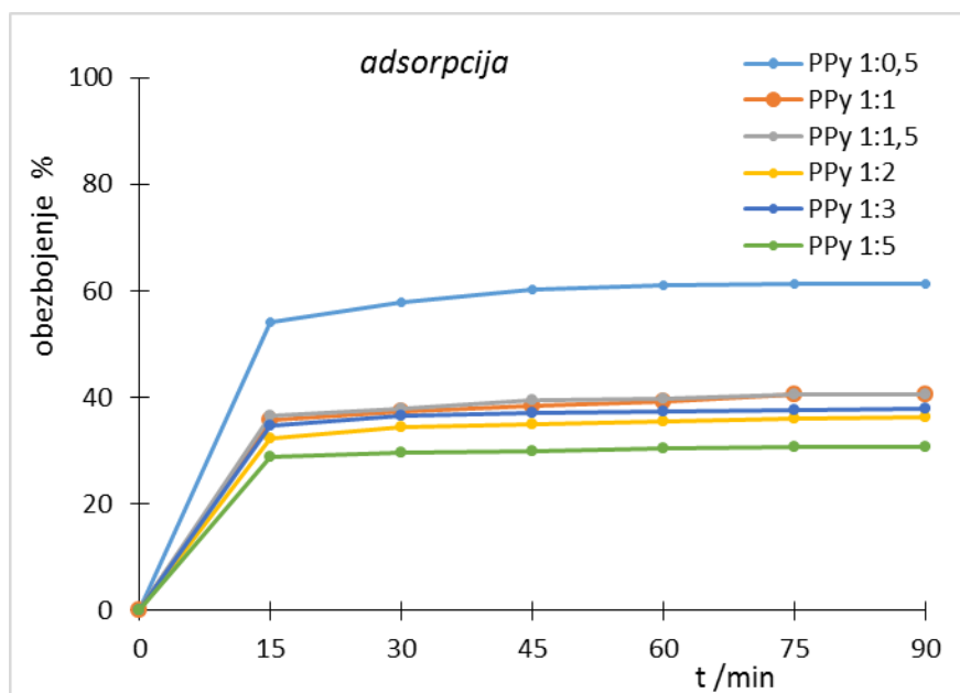
Slika 4.4.1. Postotak obezbojenja u ovisnosti o vremenu adsorpcije za uzorke PPy vodljivih polimera sintetiziranih 90 minuta
