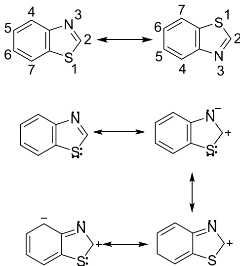
Shema 2. Rezonantne strukture benzotiazola
